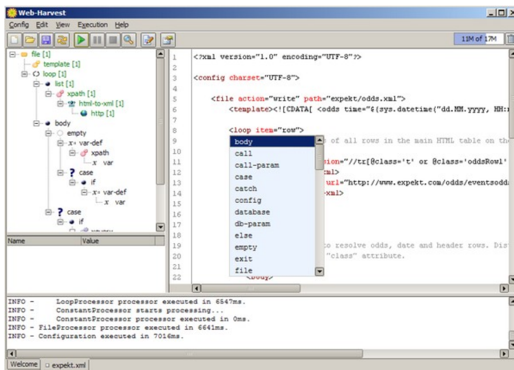
Abbildung 10: Benutzeroberfläche von WebHarvest (Nikic o. D.)
