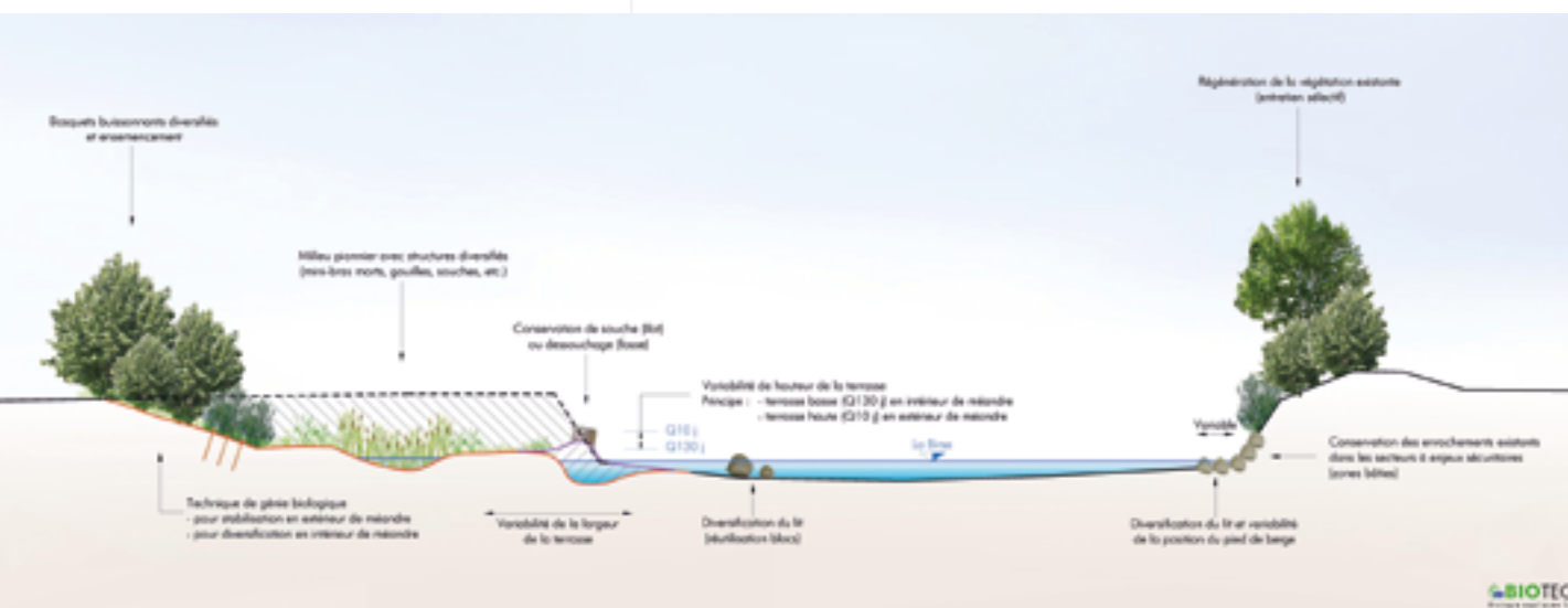
PROFIL TYPE D'AMÉNAGEMENT DU LIT DE LA BIRSE
